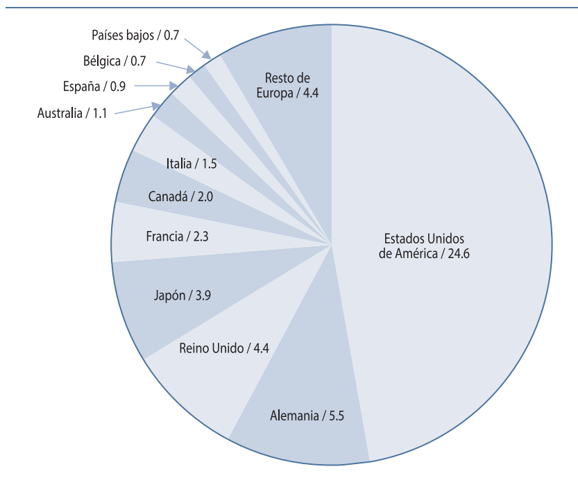
GRÁFICO 8 Contribución porcentual por país de 50% de las emisiones de dióxido de carbono en el mundo (1850–2020)
